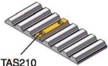
TAS210 - 适于AT10齿型, 32 mm宽, 双销, 中心距20 mm
