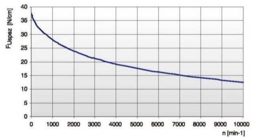
同步带齿部剪切强度/rpm
