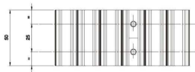
TAS158 - 适于AT20和XH齿型, 25-50-75-100 mm宽, 多销, 中心距25 mm
