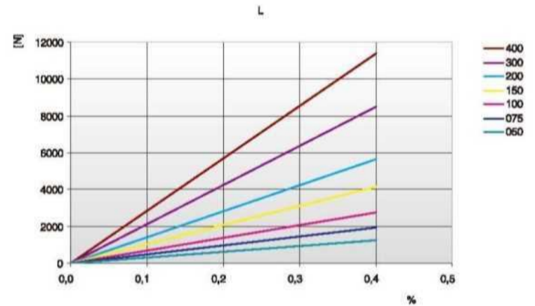
负载/延伸率 [%]
