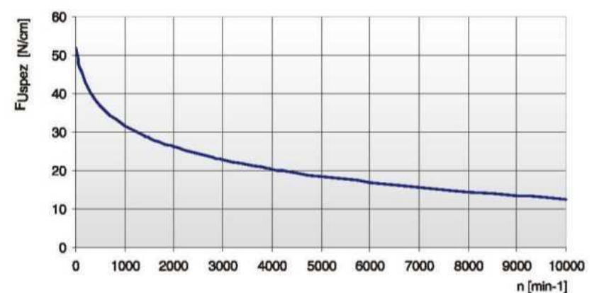
同步带齿部剪切强度/rpm
