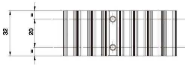
TAS210 - 适于AT10齿型, 32 mm宽, 双销, 中心距20 mm
