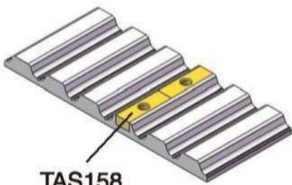
TAS158 - 适于AT20和XH齿型, 25-50-75-100 mm宽, 多销, 中心距25 mm
