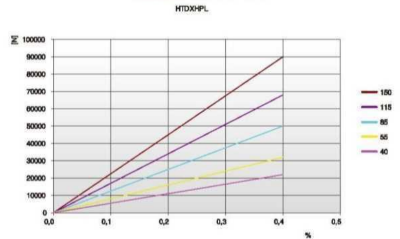
负载/延伸率 [%]
