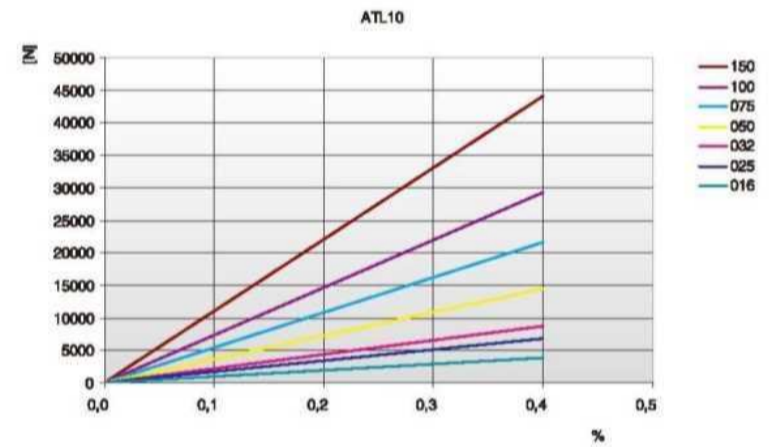
负载/延伸率 [%]
