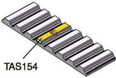
TAS154 - 适于AT10和H齿型, 25 mm宽, 单销
