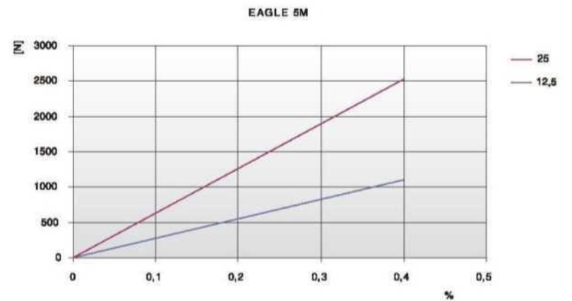
负载/延伸率 [%]
