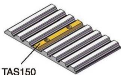
TAS150 - 适于AT10齿型, 50 mm宽, 双销, 中心距25 mm
