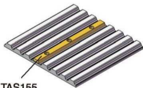
TAS155 - 适于AT10齿型, 75 mm宽, 三销, 中心距25 mm
