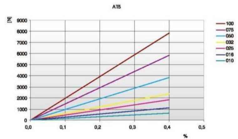
负载/延伸率 [%]
