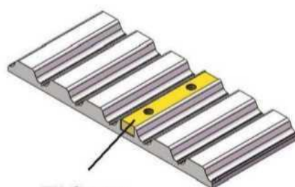
TAS142 - 适于AT20和XH齿型, 50 mm宽, 双销, 中心距25 mm
