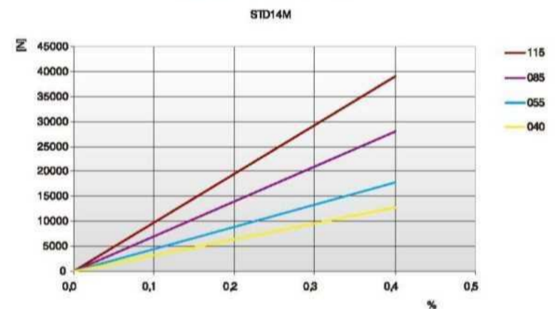
负载/延伸率 [%]
