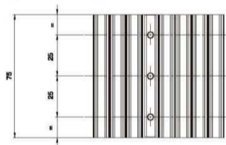
TAS155 - 适于AT10齿型, 75 mm宽, 三销, 中心距25 mm
