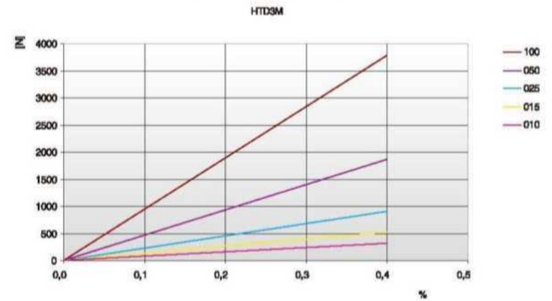
负载/延伸率 [%]
