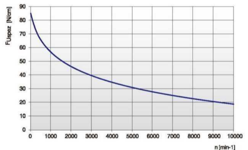
同步带齿部剪切强度/rpm
