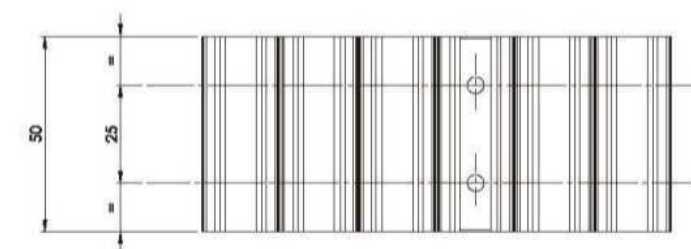
TAS142 - 适于AT20和XH齿型, 50 mm宽, 双销, 中心距25 mm
