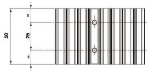
TAS150 - 适于AT10齿型, 50 mm宽, 双销, 中心距25 mm
