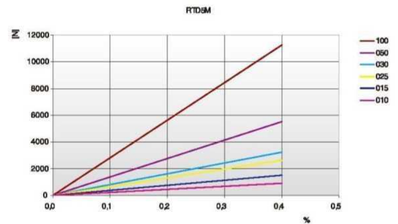
负载/延伸率 [%]
