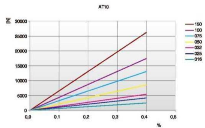
负载/延伸率 [%]
