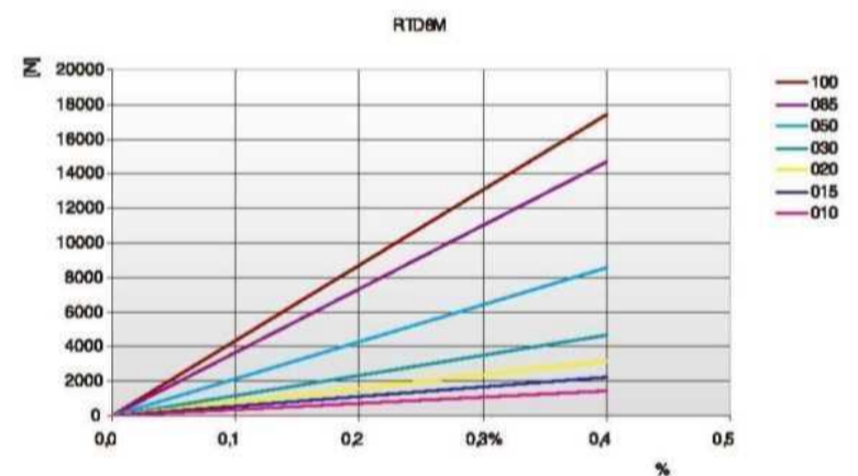
负载/延伸率 [%]
